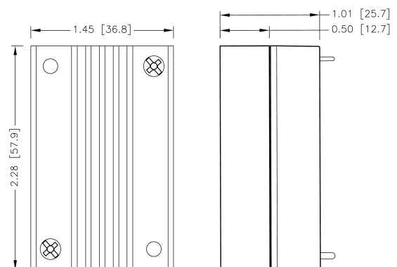
QAE60-□□S□□U -HS3 7G-0032B-F
